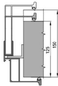
S3 толщина стены проёма от 125 до 150 мм
