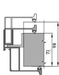
S1 толщина стены проёма от 73 до 98 мм
