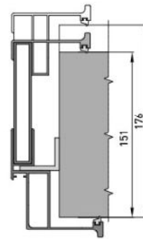
S4 толщина стены проёма от 151 до 176 мм
