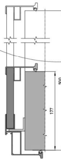
S177-S500 толщина стены проёма от 177 до 900 мм
