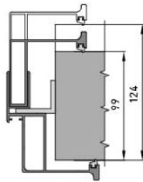
S2 толщина стены проёма от 99 до 124 мм
